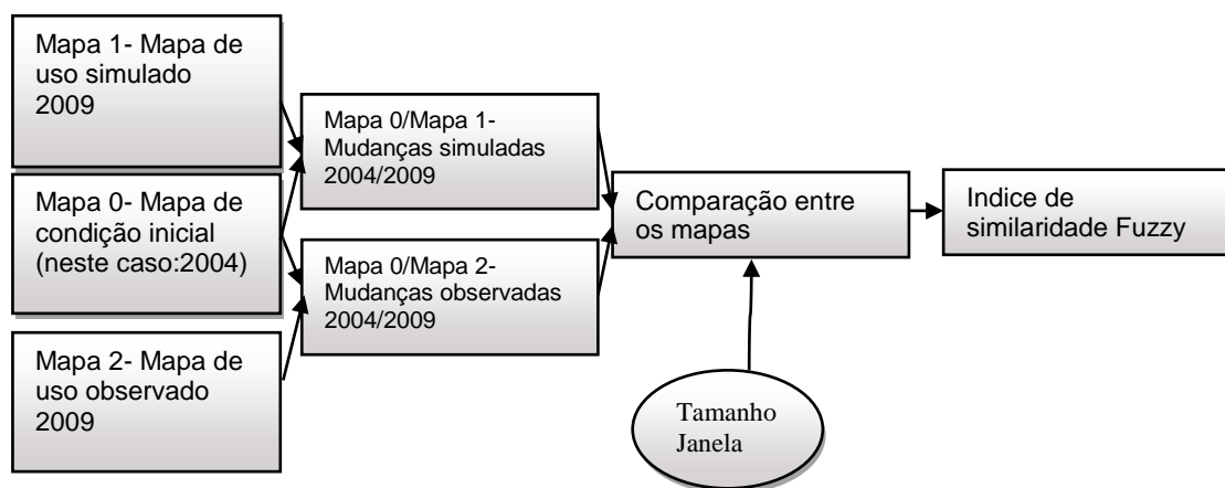
Figura 29. Fluxograma dos processos do modelo desenvolvido no DINAMICA-EGO para calcular o índice de similaridade.
